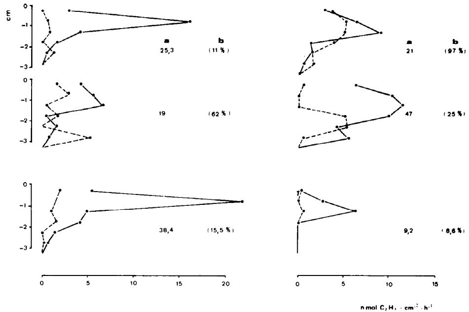
FIG. 1. - Variations verticales de l'ARA mesurée à la lumière (● — ●) et à l'obscurité (● - - ●) ; (a) : activité totale à la lumière (nmol C 2 H 4 .cm -2 .h -2 ), (b) : activité totale à l'obscurité exprimée en % de l'activité totale à la lumière.
