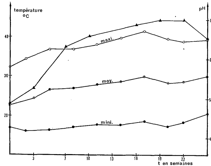
FIG. 2. — Variations du pH de l'horizon 0-1 cm : \blacktriangle — \blacktriangle et de la température ambiante journalière (moyenne sur 21 jours : température maximale : \circ — \circ ; température moyenne : \square — \square ; température minimale : \bullet — \bullet ).
